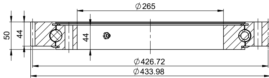
VIEW A-A
