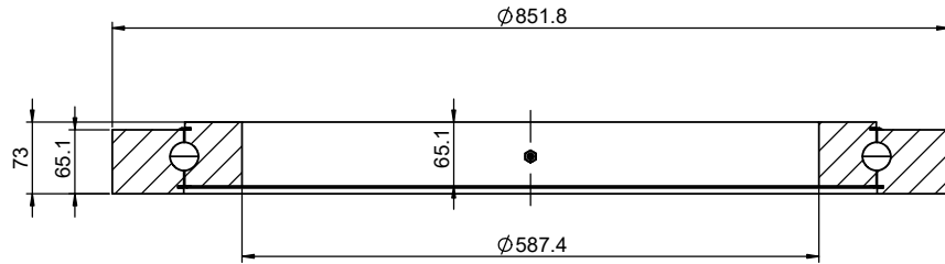
VIEW A-A
