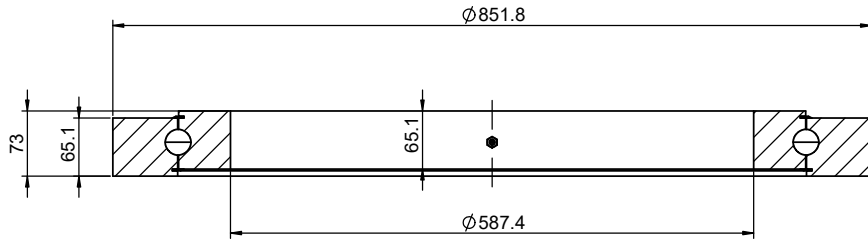
VIEW A-A
