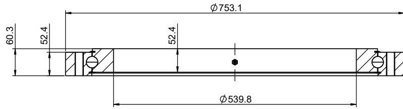
VIEW A-A
